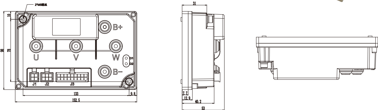
产品尺寸图
