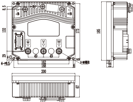
LC080350-**N
