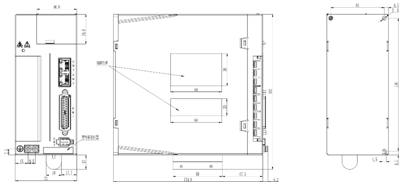
FS3210/FS3215- ATE 安装尺寸图
