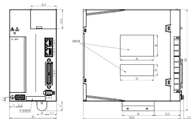
FS3409/FS3413-ATE 安装尺寸图
