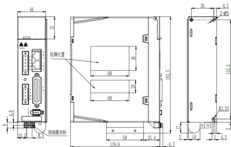
FS3201/FS3202/FS3204- ATE 安装尺寸图
