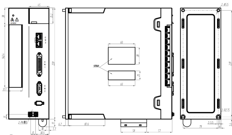
FS3417/FS3425-ATE 安装尺寸图
