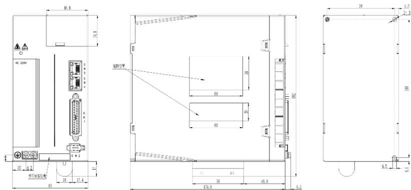
FS3220- ATE 安装尺寸图
