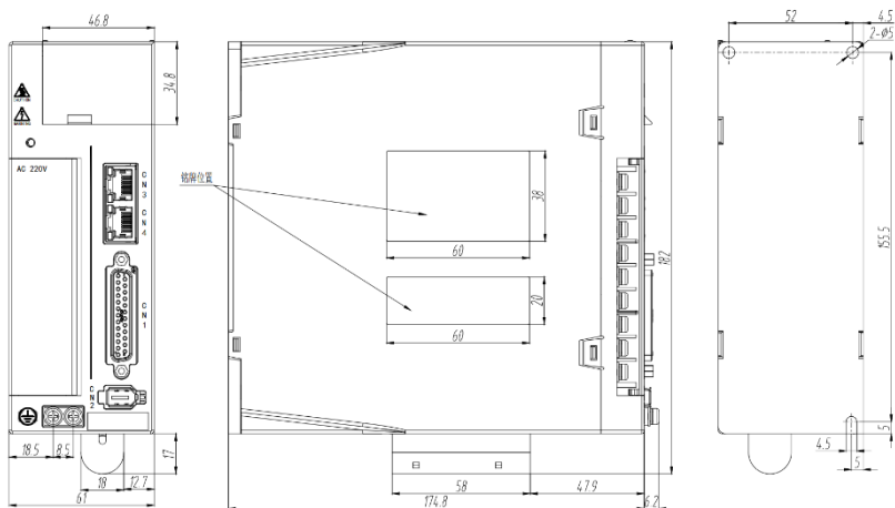
FS3404-ATE 安装尺寸图
