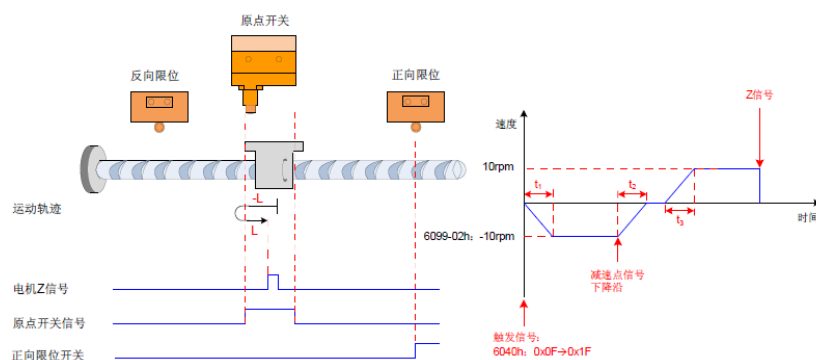
图 4-16 6098h=8 且减速点信号有效模式③
