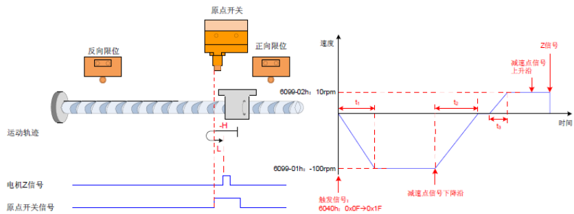
图 4-9 6098h=4 且减速点信号有效模式②
