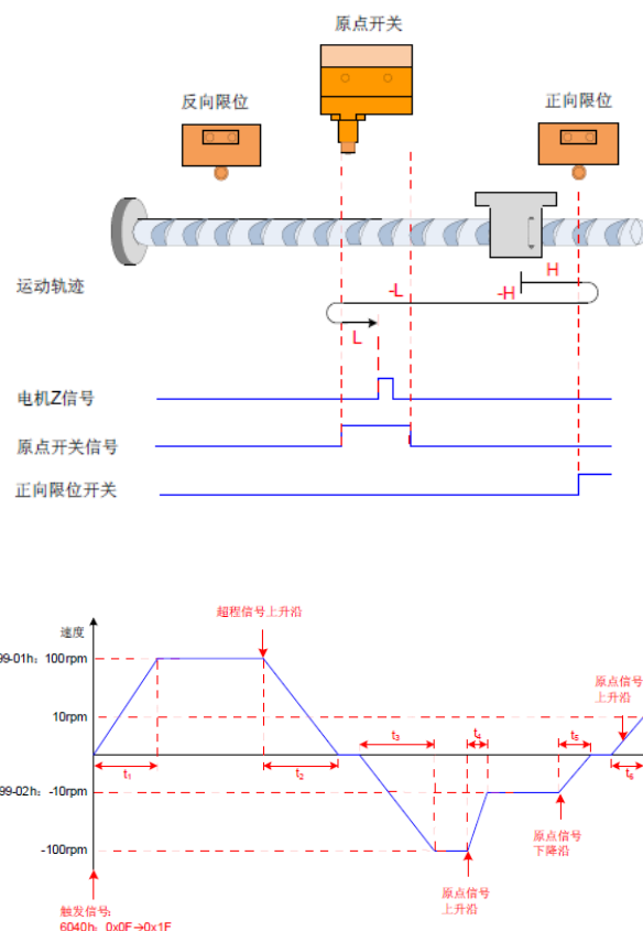
图 4-15 6098h=8 且减速点信号无效，遇到正限位开关模式②
