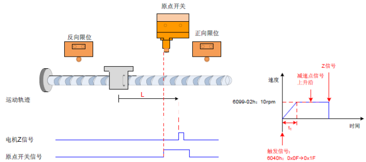
图 4-8 6098h=4 且减速点信号无效模式①
