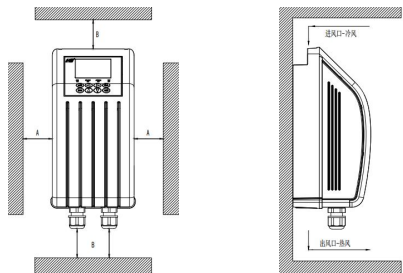
图 2-2：安装示意图
