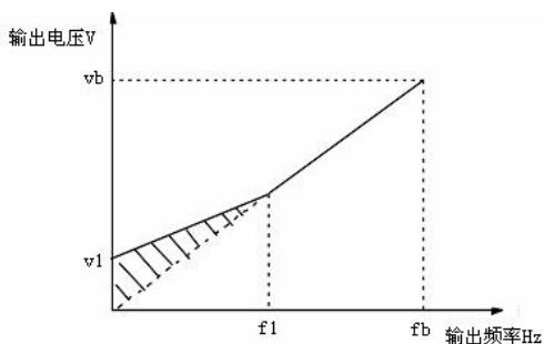
图 4-2: 转矩提升示意图
