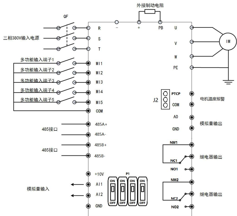
图 2-3：VD600 接线示意图
