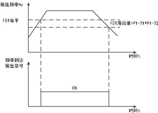
图 4-13: FDT 电平检测示意图
