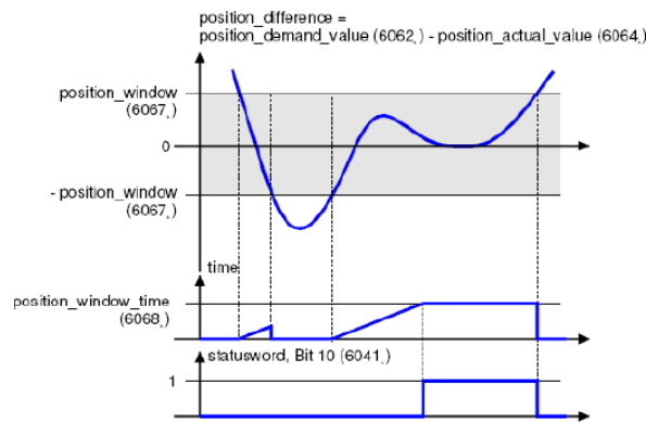
图 4-20 位置到达功能描述
