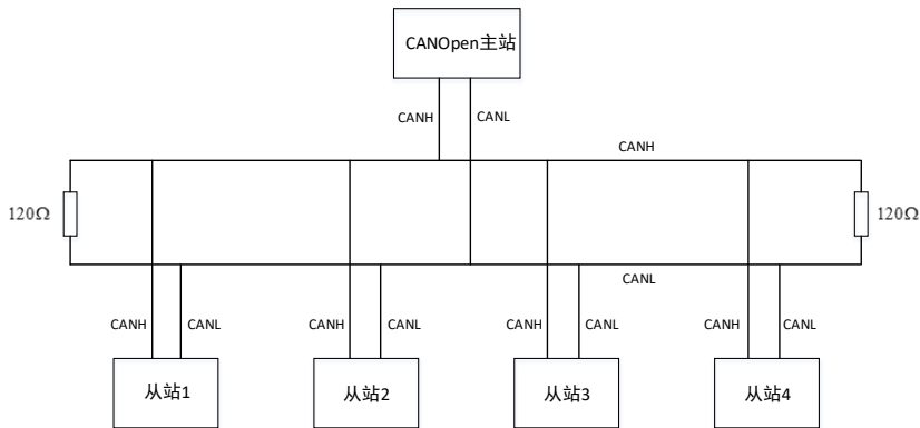
图 2-2 CANOpen 通信网络拓扑结构图
