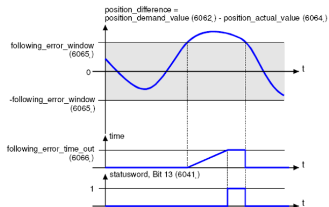
图 4-18 跟随误差功能描述
