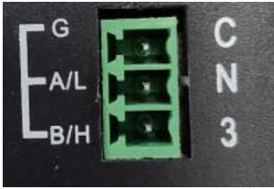
图 2-1 DHE 系列通讯口图片
