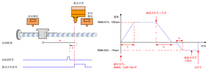
图 4-6 6098h=3 且减速点信号无效模式①
