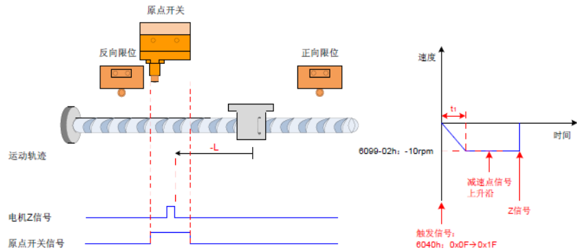
图 4-12 6098h=6 且减速点信号无效模式①
