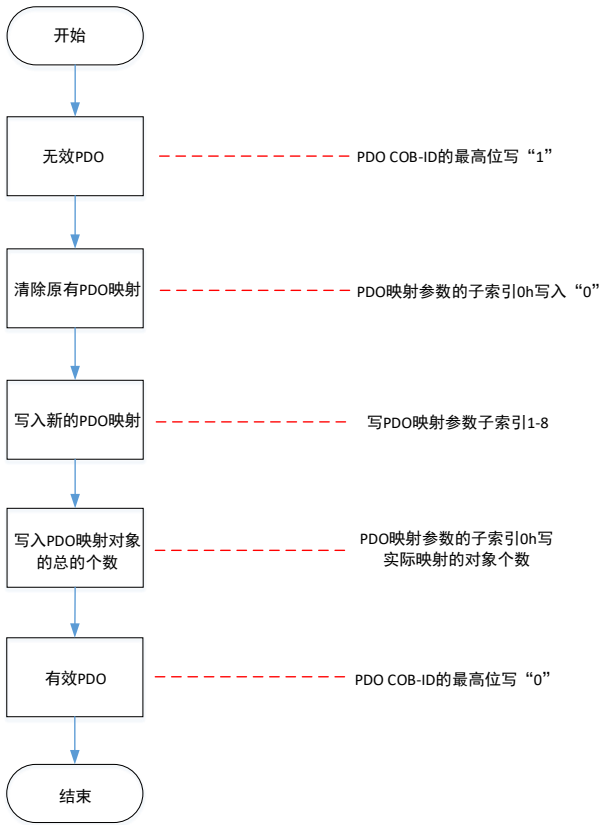
图 3-3 PDO 映射配置流程图
