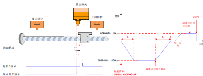
图 4-9 6098h=4 且减速点信号有效模式②
