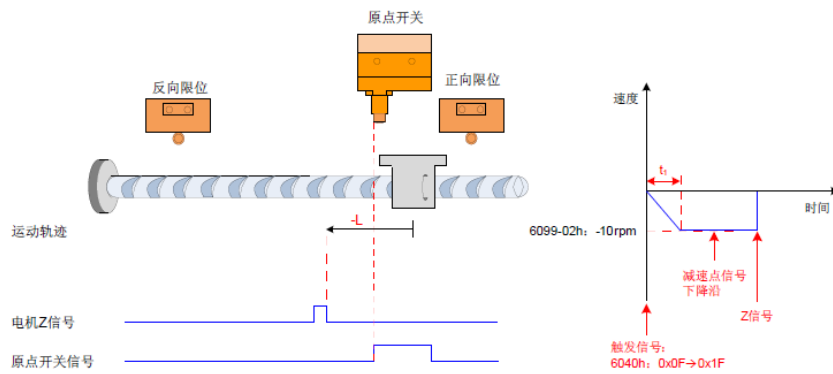
图 4-7 6098h=3 且减速点信号有效模式②
