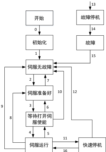
图 4-1 CiA402 状态机切换图
