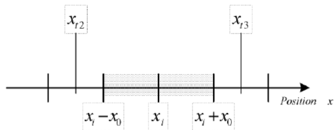
图 4-3 跟随误差举例
