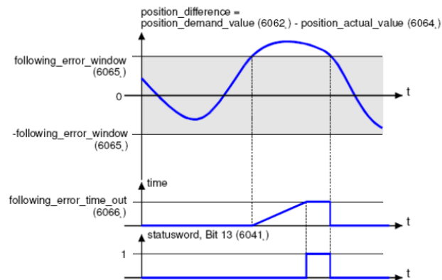
图 4-2 跟随误差功能描述
