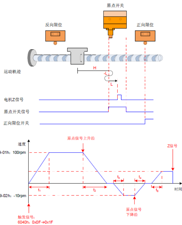
图 4-14 6098h=8 且减速点信号无效，遇到正限位开关模式②
