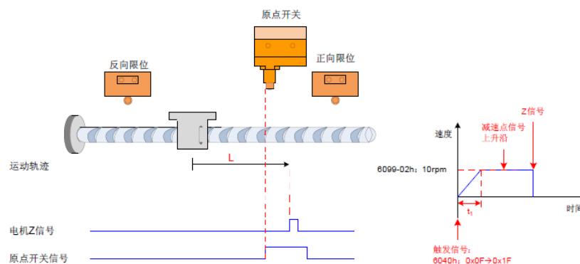
图 4-8 6098h=4 且减速点信号无效模式①
